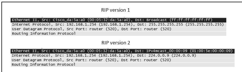
Rysunek 5.11. Adresowanie w protokole RIP
