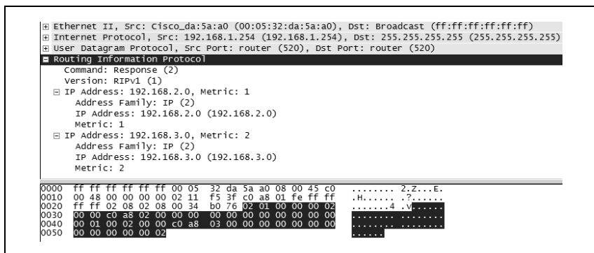
Rysunek 5.2. Pakiet protokołu RIPv1
