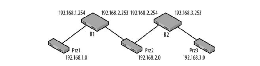
Rysunek 5.28. Topologia do ćwiczenia 1.
