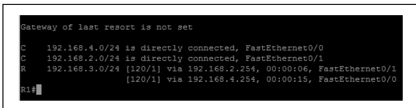
Rysunek 5.24. Tablica trasowania routera R1
